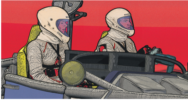
Mars
